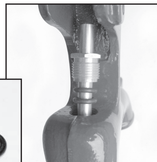
Écrou d'emballage
